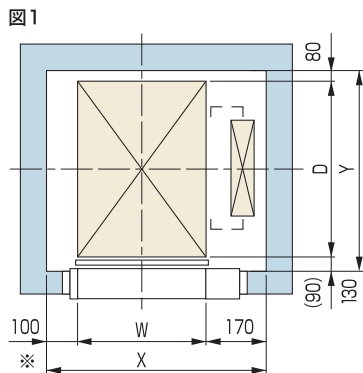
●昇降路平面図
