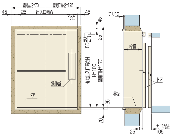
●テーブルタイプ寸法表
