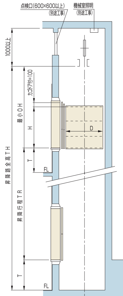
●昇降路断面図
